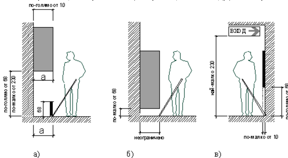
Фиг. 6. Ориентация на решетките, покриващи шахти и други отвори
