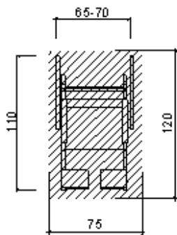
Свободна площ за инвалидна количка
