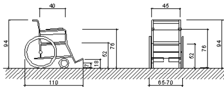
Размери на инвалидна количка
