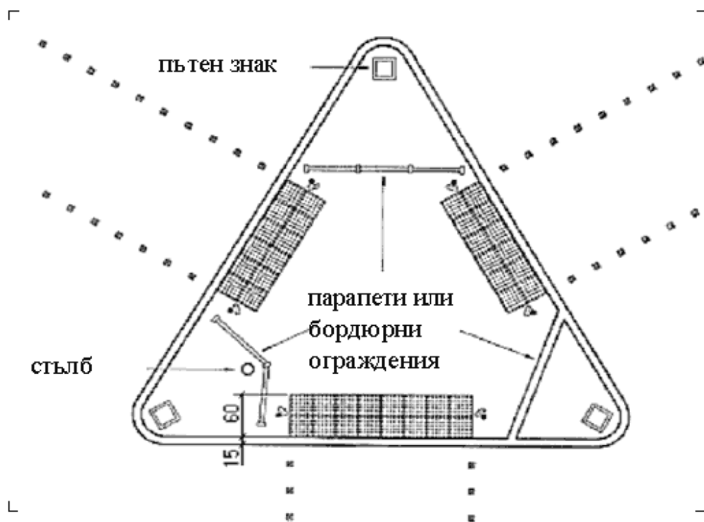
Фиг. 12. Разполагане на тактилни плочи на остров с предпазна ограда
