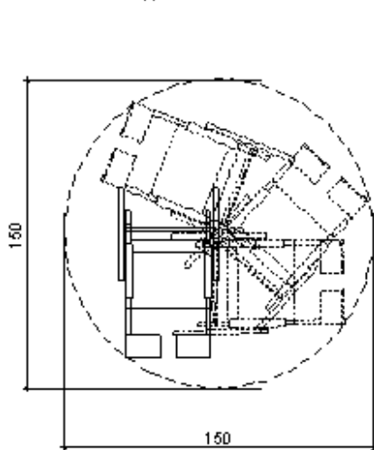
Свободна площ за инвалидна количка
