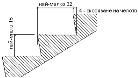
Фиг. 13. Разполагане на тактилни плочи на триъгълен остров
