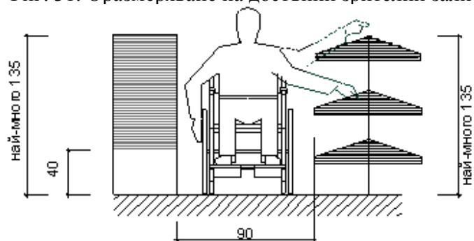
Фиг. 31. Оразмеряване на достъпни зрителни зали
