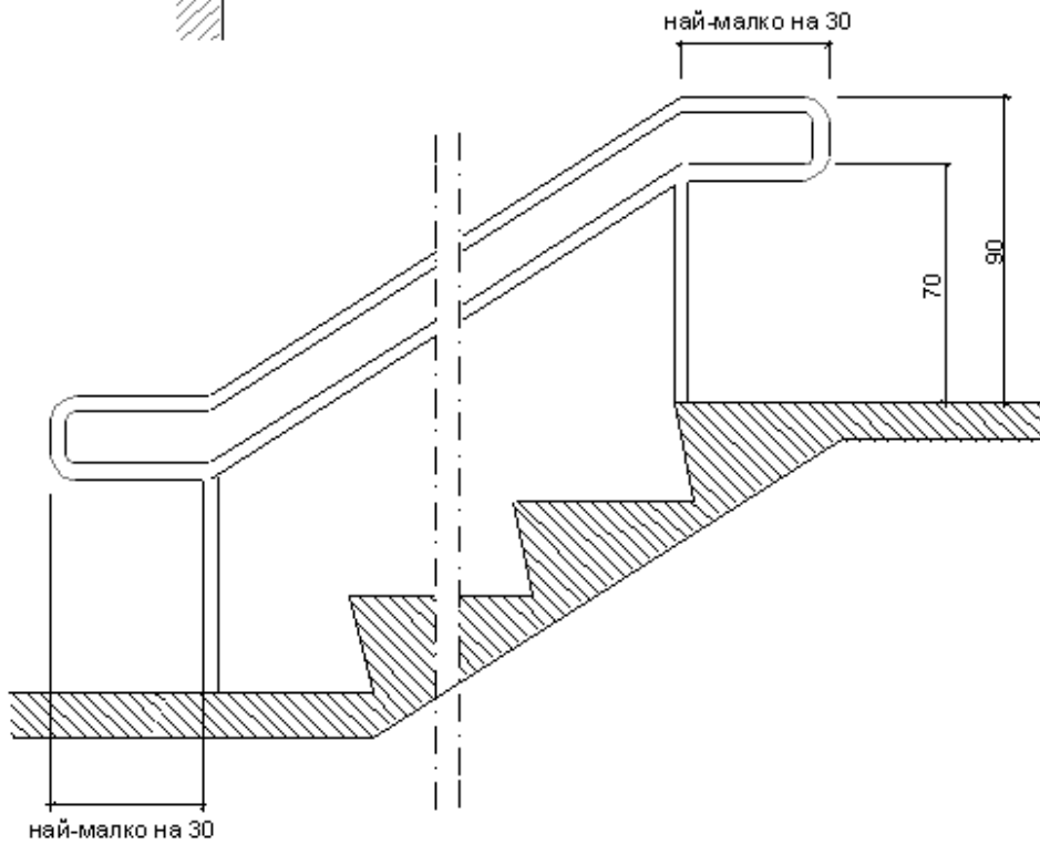
б) двоен парапет
